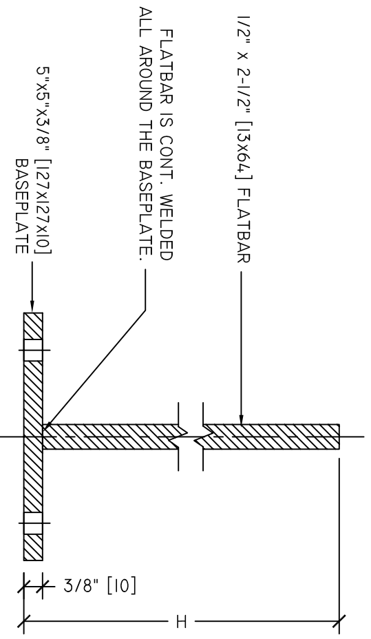
ELEV
